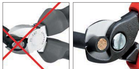
D 15 самораскрывающиеся, с раскрывающей пружинкой в головной части self-opening spring in head
