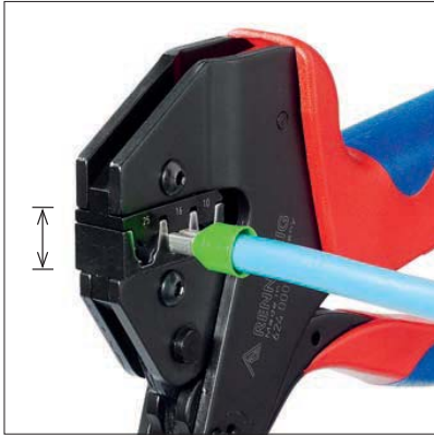
Ширина раствора 12 мм Opening width 12 mm
