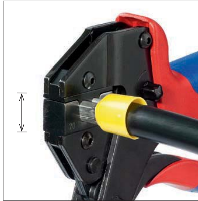
Ширина раствора 16 мм Opening width 16 mm
