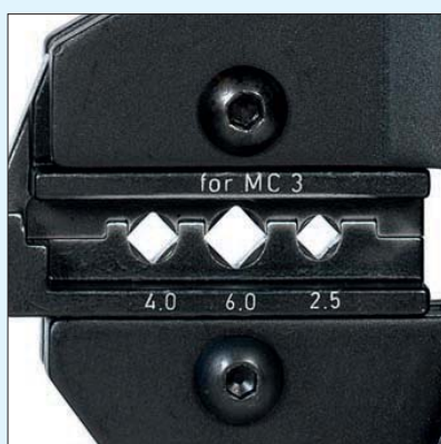
Опрессовочная плашка, сменная (пример использования: с разъемом MC 3)
